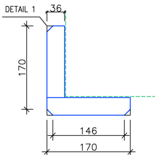
LÕIGE 1-1 M 1:5
