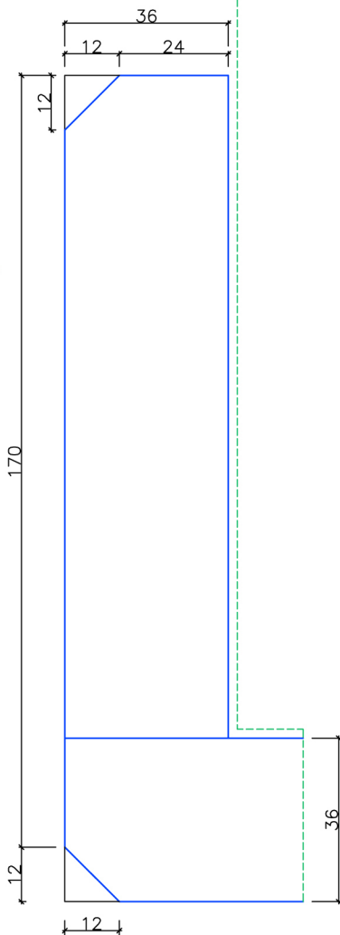
DETAIL 1 M 1:1
