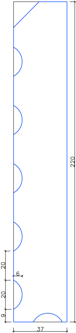
DETAIL 4 M 1:1
