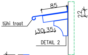
LÕIGE 2-2 M 1:5
