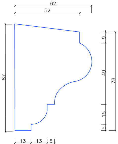
DETAIL 2 M 1:1
