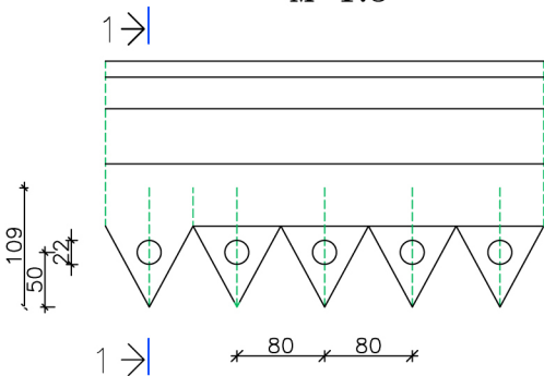
VAADE M 1:5
