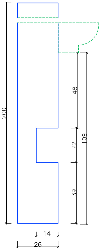
DETAIL 1 M 1:1
