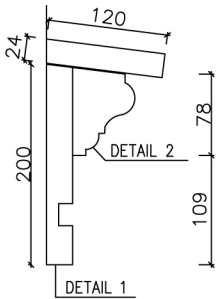
LÕIGE 1-1 M 1:5
