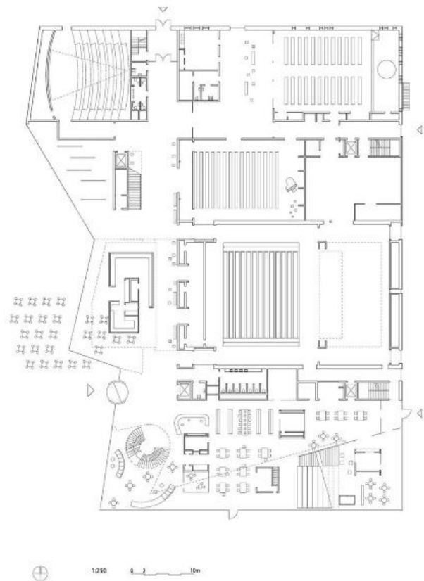
Hoone plaan
