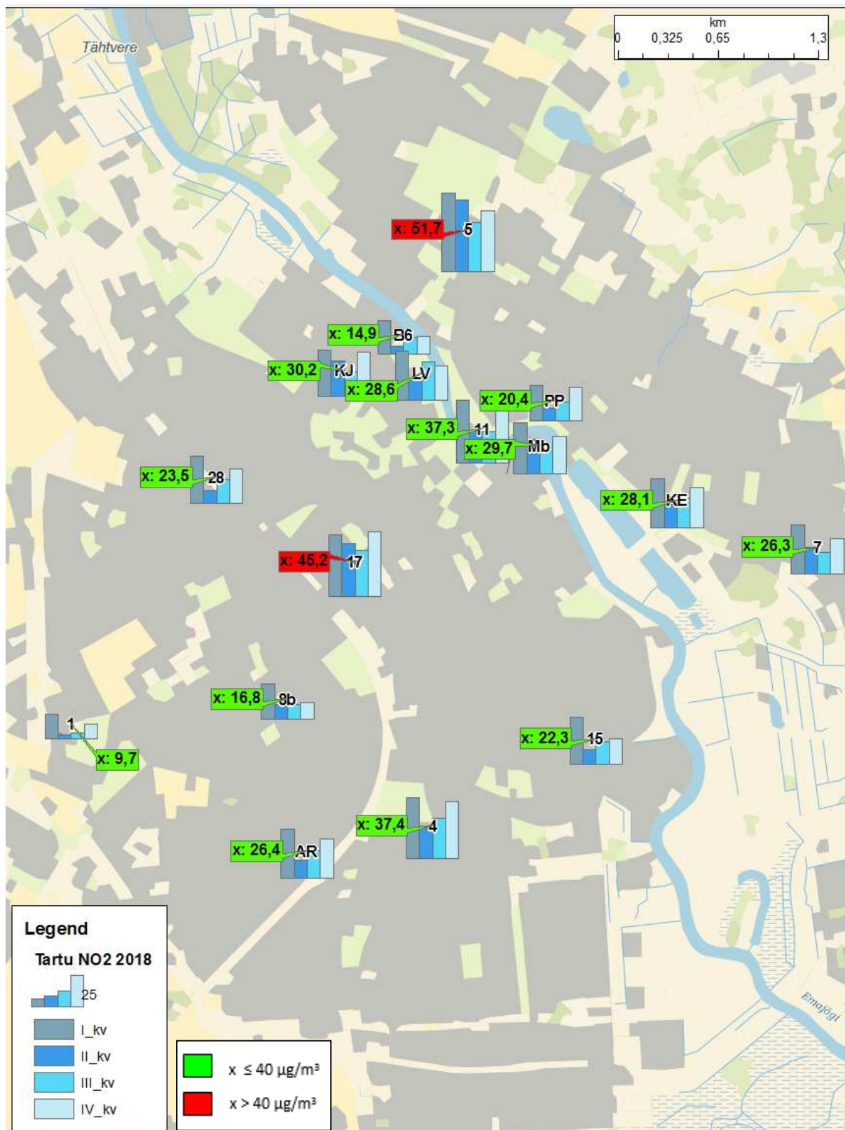
Joonis 2. Tartu linna 2018. aasta välisõhu saasteaine NO 2 kontsentratsioonid I, II, III ja IV kvartalis, 2018. aasta keskmine x (Nr diagrammil on seirejaama tähis)
