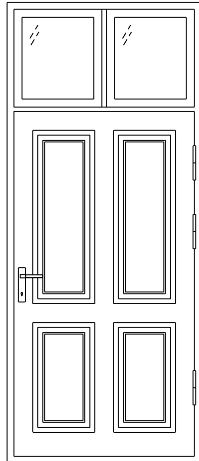
Vaade seest m1:20
