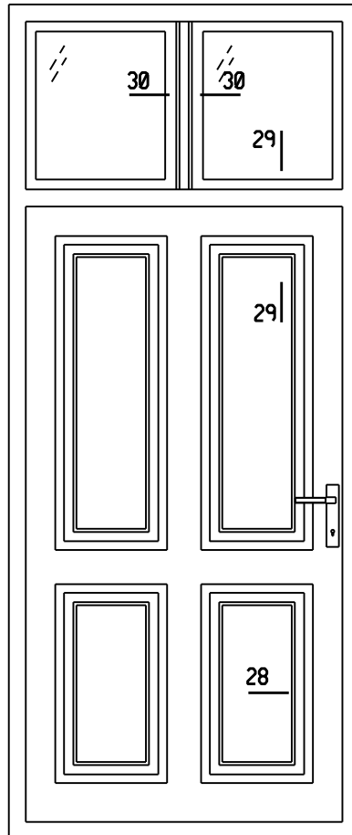
Vaade väljast m1:20
