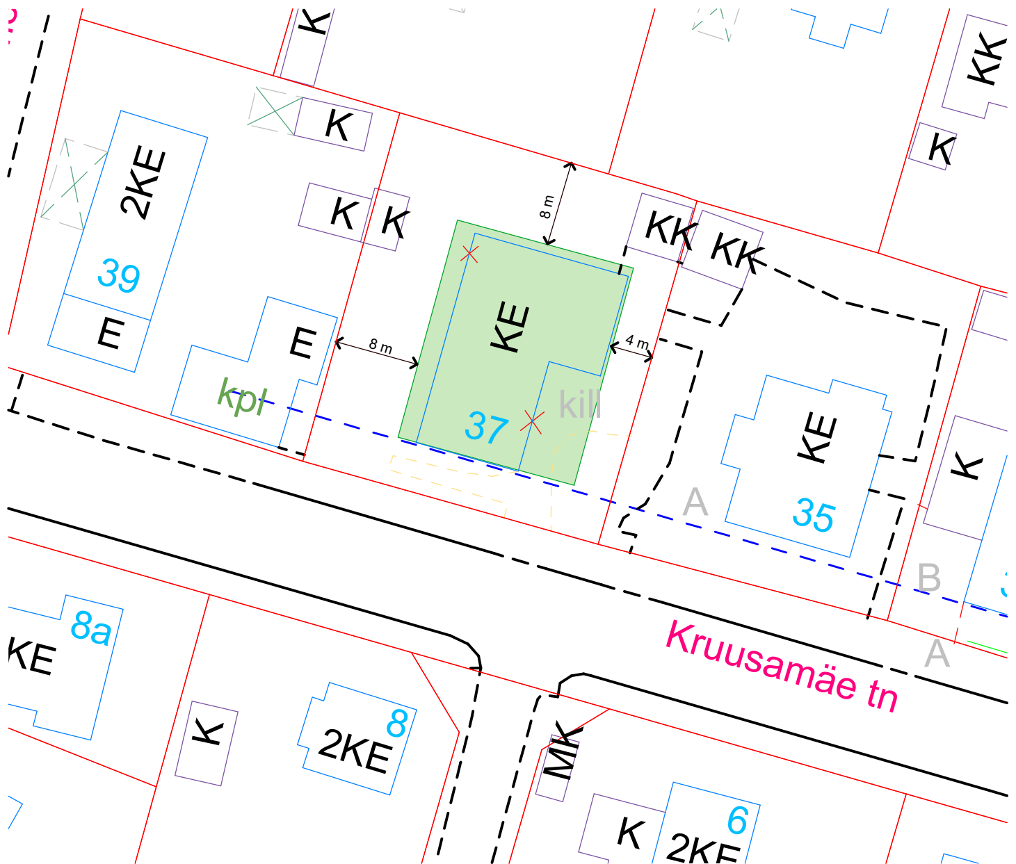
Lisa. Kruusamäe tn 37 ehitusala skeem PTH-24-012
