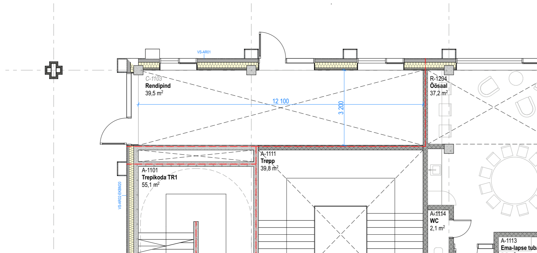
Vabaduse puistee kohviku ruumid 1. korrusel
