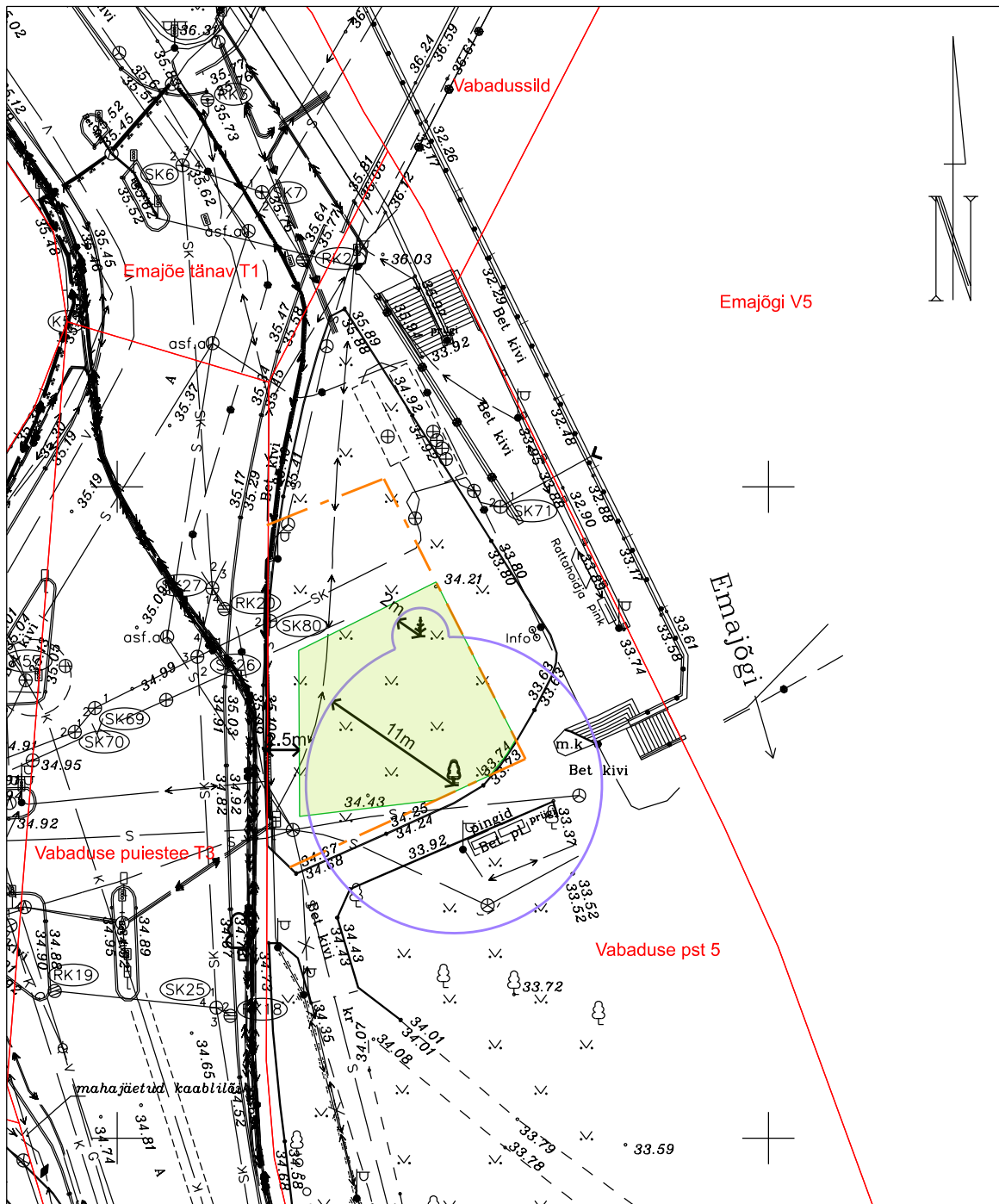
Lisa. Vabaduse pst 5 ehitusala skeem PTH-23-053
